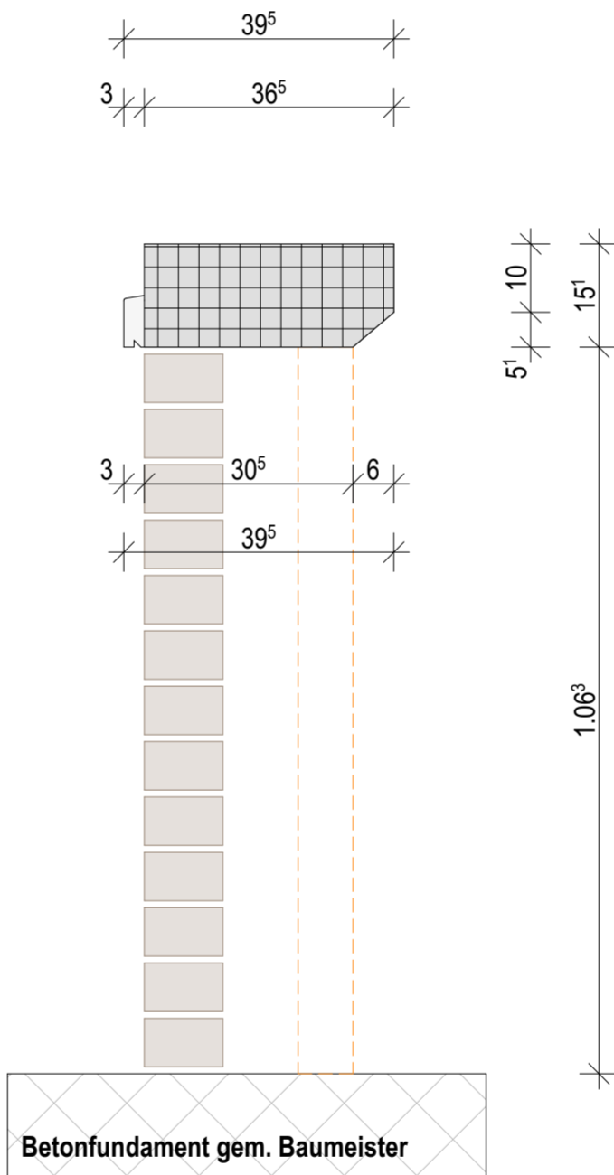
Schnitt A
