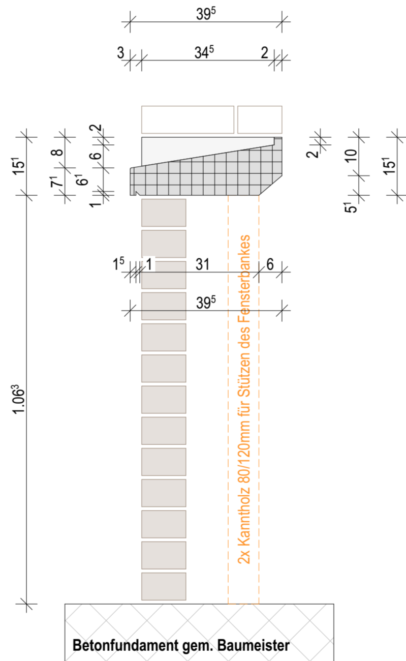
Schnitt A
